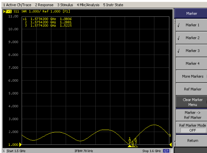
VSWR
